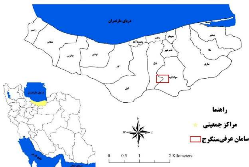
شکل ۱: موقعیت جغرافیایی منطقه سنگر
