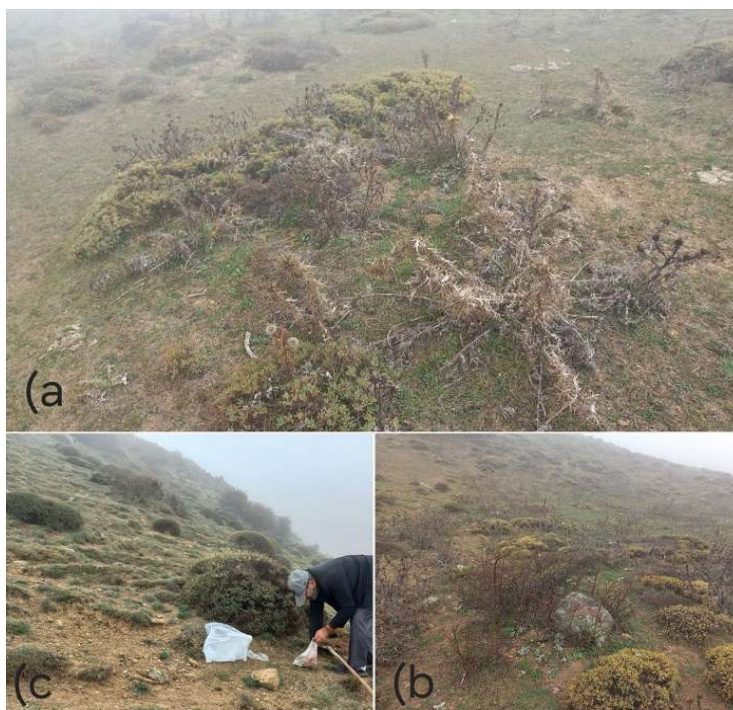
شکل ۲: نمایی از سه دامنه شمال، شرق و غرب منطقه (به ترتیب a، b و c)
